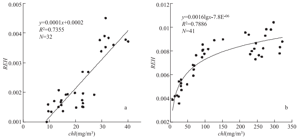
图 4 REH 与叶绿素的关系: 水库(a); 芙蓉湖(b)
